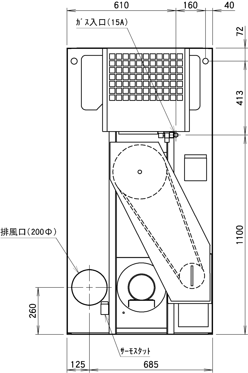
VG130C 外観図
