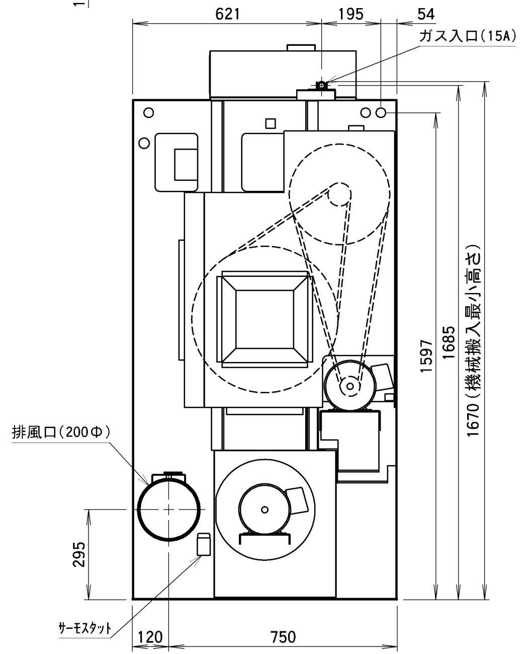
VG200C 外観図
