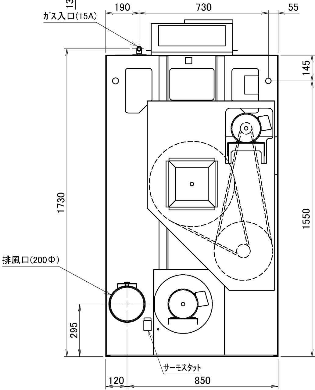
VG251C 外観図
