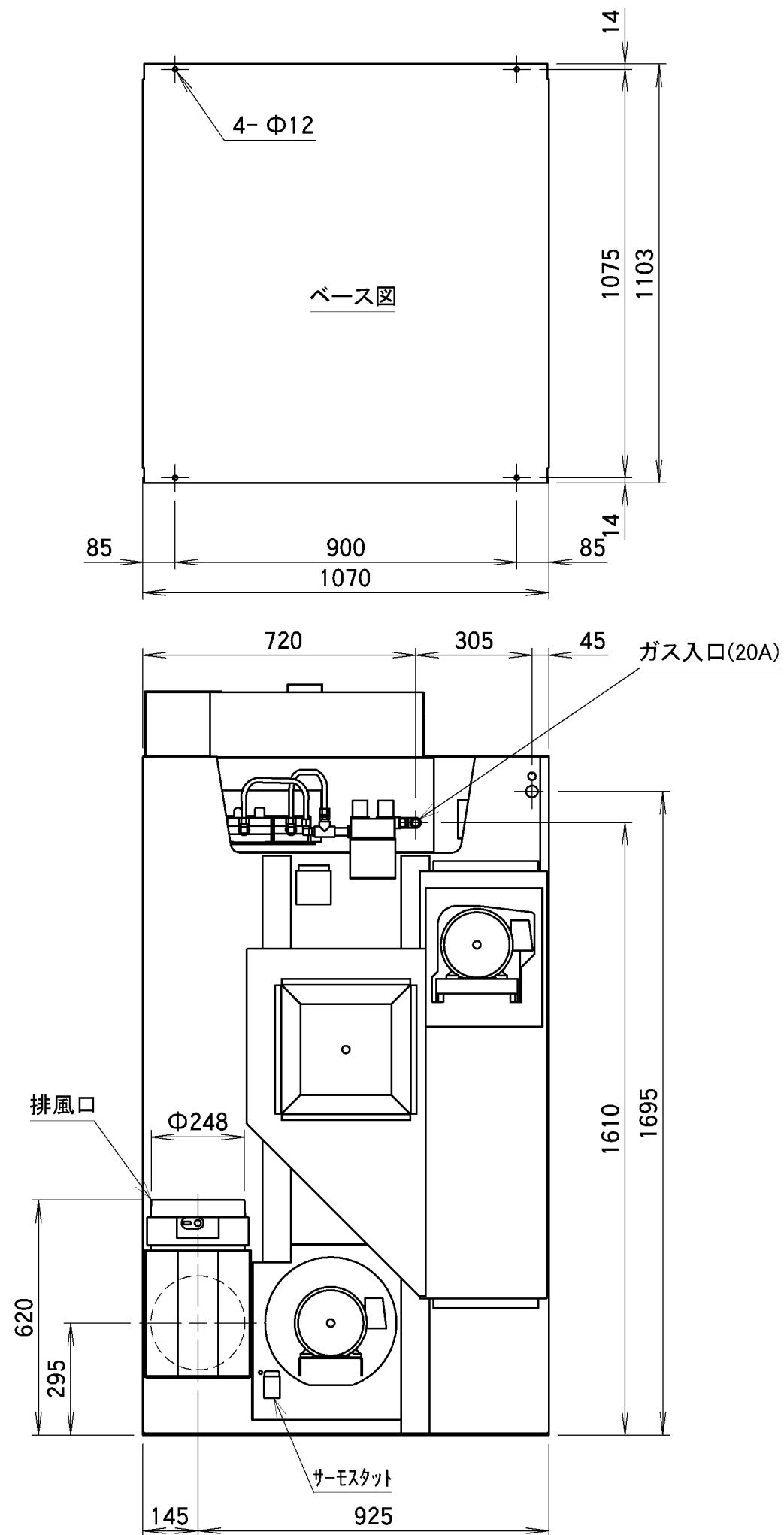
VG350C 外観図
