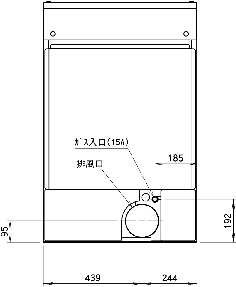
VG90C外観図
