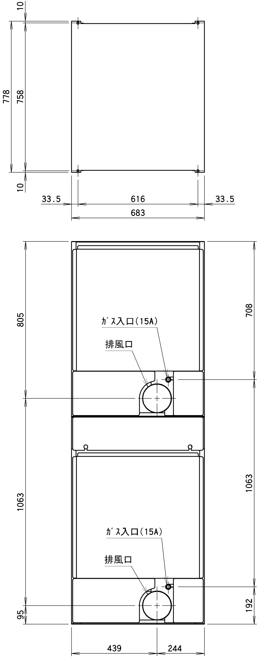
VG90CW外観図
