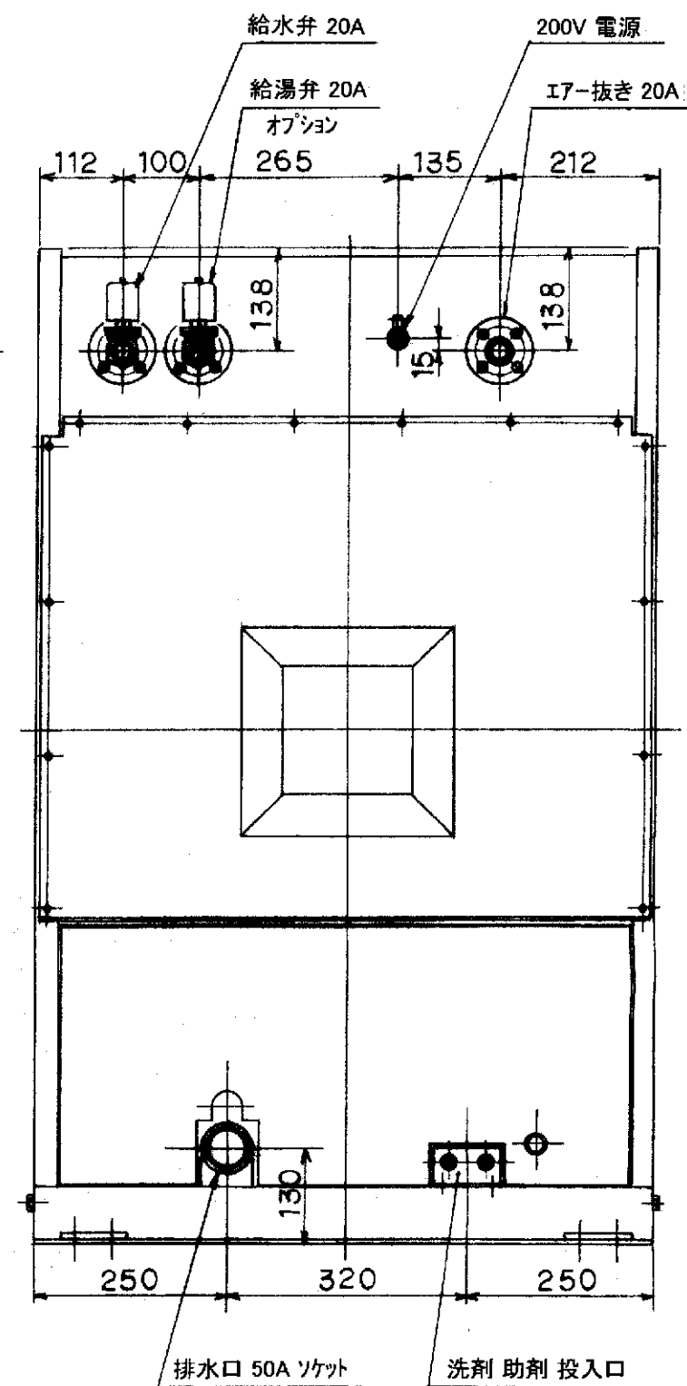
WN130CL 外觀圖
