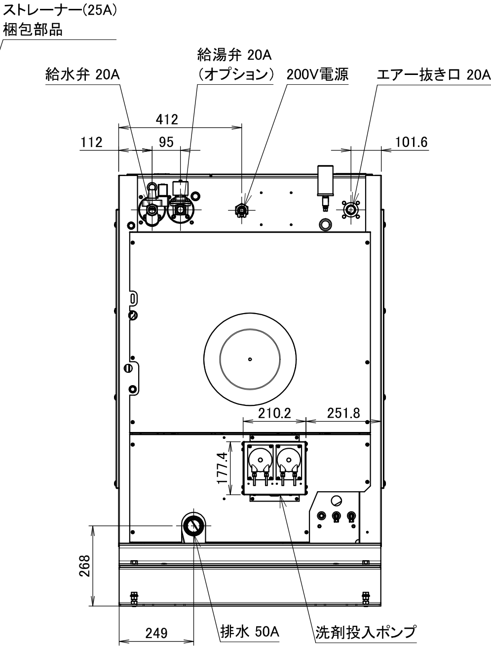
WN131CS 外観図
