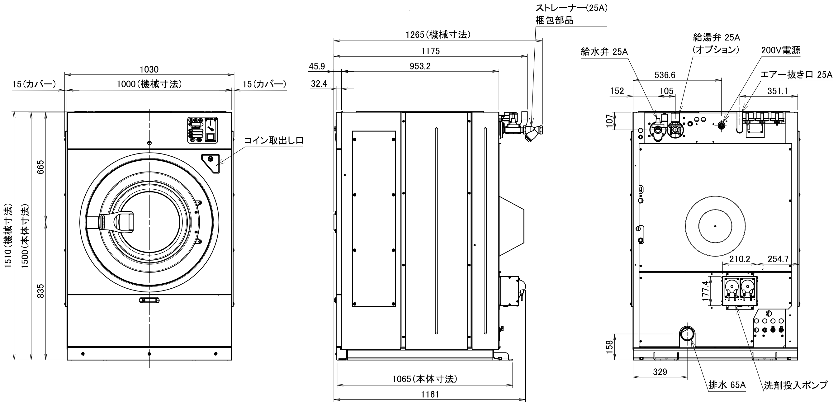
WN231CS 外観図
