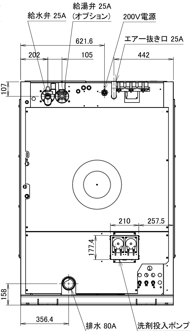
WN281CS 外観図
