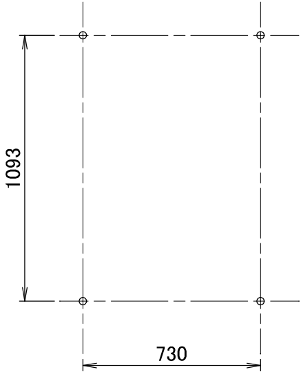
(アンカーボルト位置)
