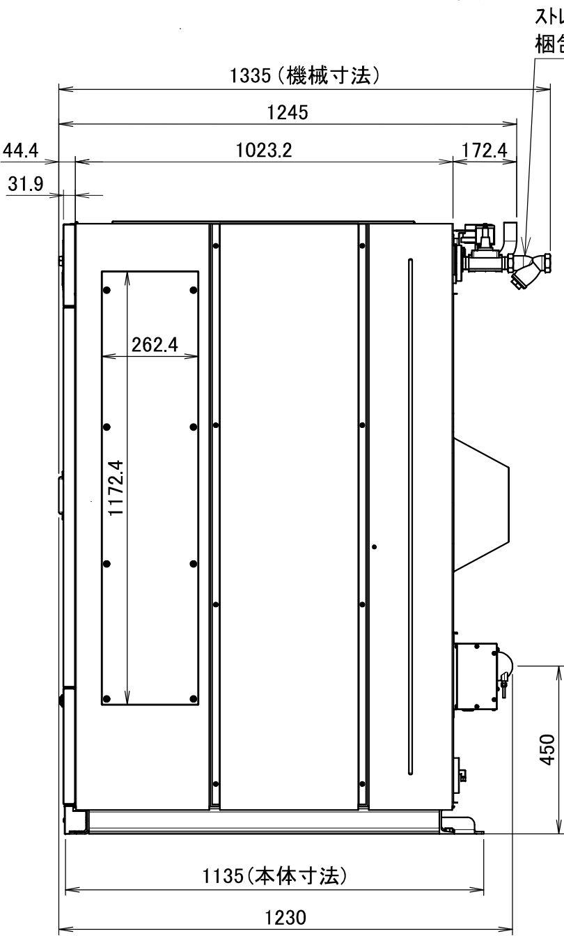
(アンカーボルト位置)
